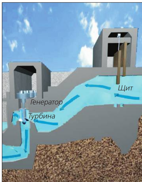
Рис. 45. Гидроэлектростанция
