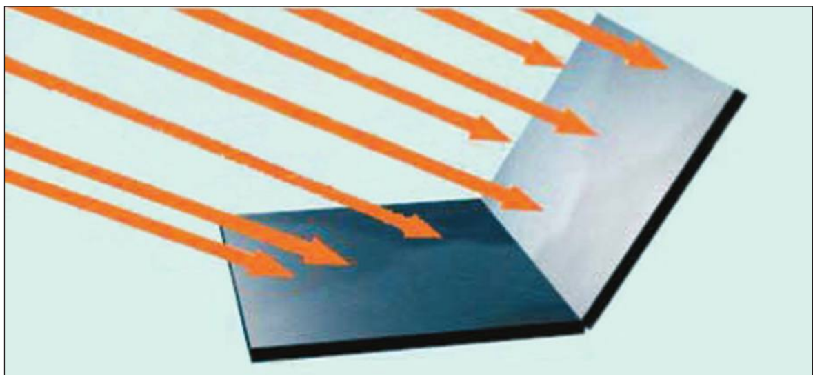
Рис. 75. Нагревание солнечными лучами пластин, расположенных под разными углами
