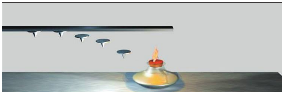
Рис. 23. Опыт, доказывающий теплопроводность металлической пластинки (кнопки приклеены к пластине легкоплавким веществом)
