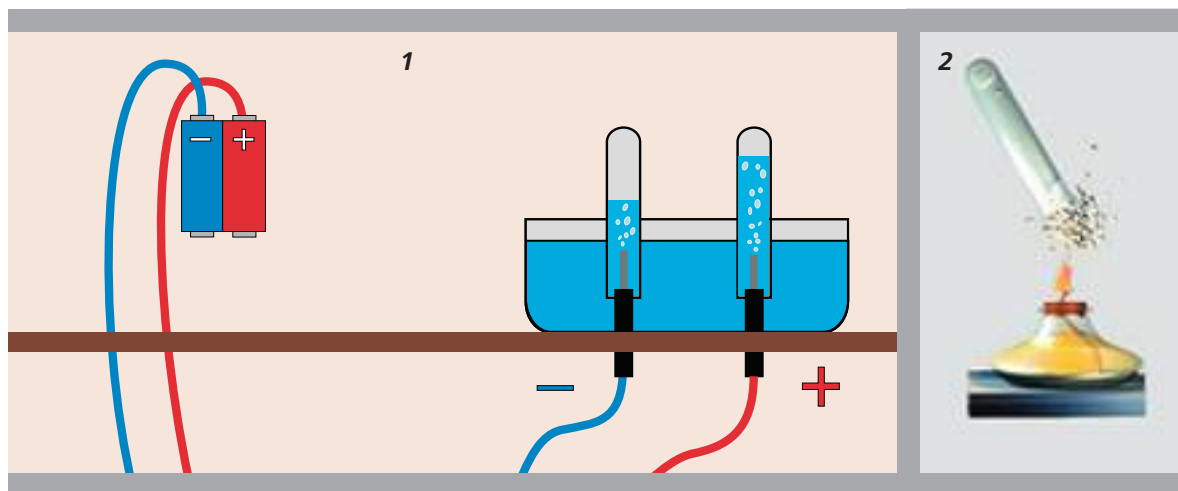
Рис. 37. Разложение воды электрическим током (1); взрыв смеси водорода с кислородом и образование воды (2)
